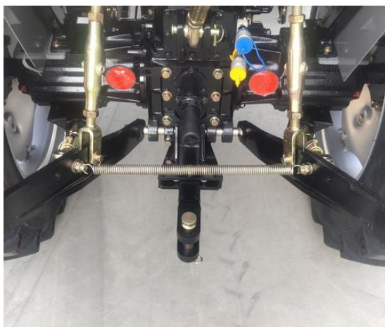
Пружина на тягах навісного механізму для зниження вібрації
